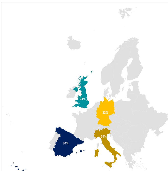
Répartition géographique 30/09/2024 (en % de la valeur vénale HD)
